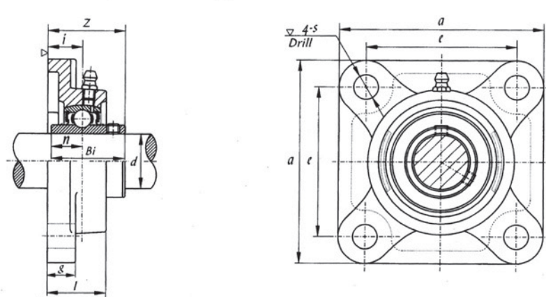
UCFX00 (medium-duty)
