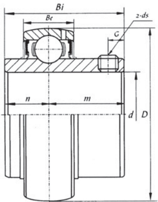
UC 200 (normal-duty)
