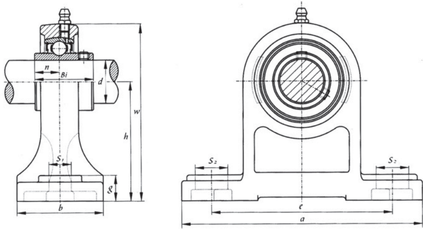
UCPH 200 (normal-duty)
