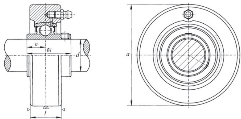
UCC 200 (normal-duty)
