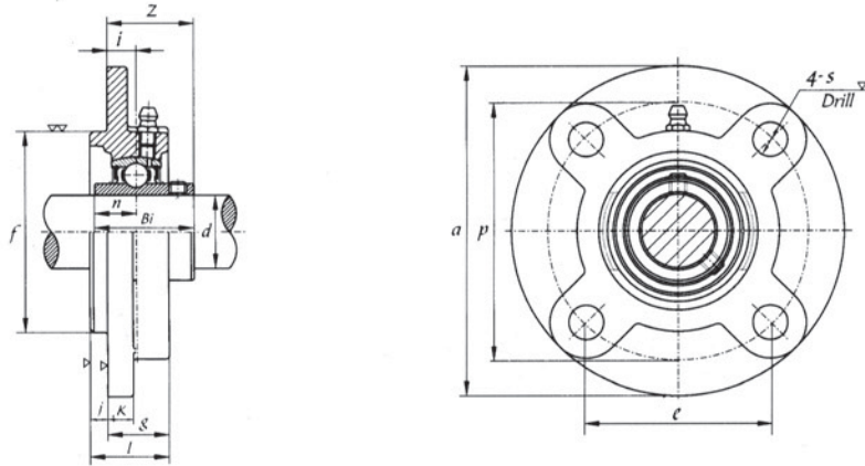
UCFC 200 (normal-duty)
